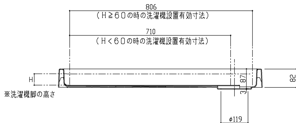
断面A-A
